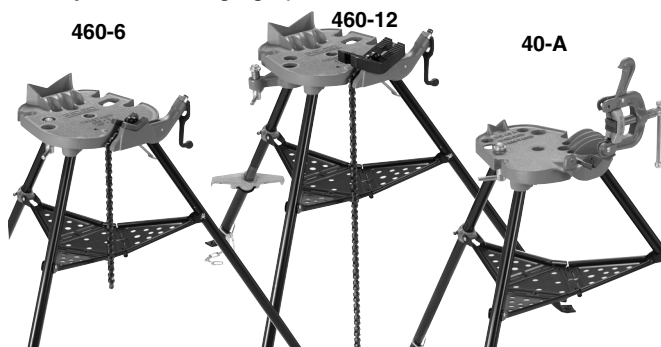
Figure 1 – Etau à tubes sur trépied RIDGID TRISTAND
